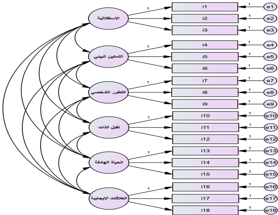
شكل رقم (1): مخرجات برنامج Amos للنموذج المختبر بست عوامل للرفاه النفسي
