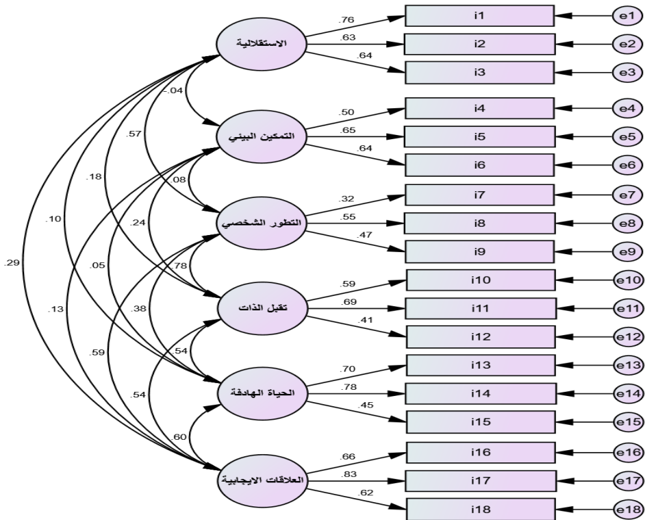
شكل رقم (02): مخرجات برنامج Amos للنموذج المختبريست عوامل للرفاه النفسي جدول رقم (1): تشبع المؤشرات المقاسة على أبعادها الفرعية للنموذج المختبريست عوامل للرفاه النفسي
