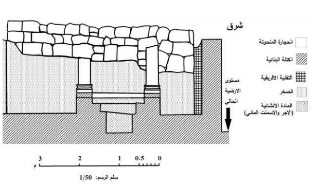
المقطع 01: يمثل مقطع غرفة التعميد الأول في تيديس. عن: فورالي، حميدة، أوت 2017م.
