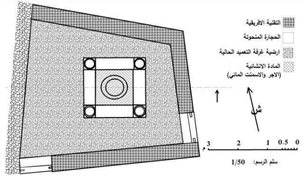
المخطط 03: يمثل مخطط غرفة التعميد الأول في تيديس. عن: فورالي، حميدة، أوت 2017م.
